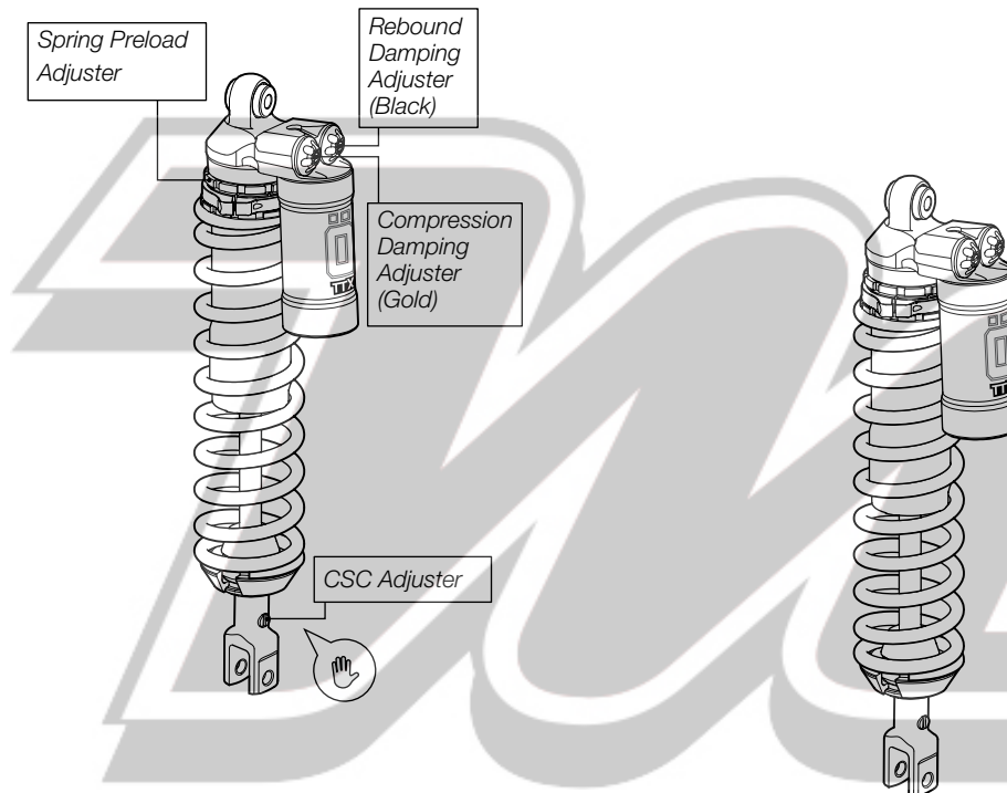
Öhlins Shock Absorber TTX44 KT 994
